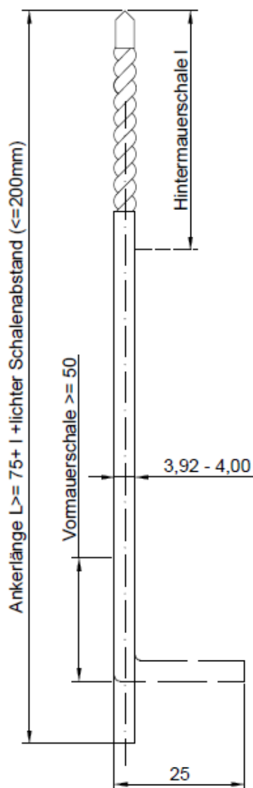
"L-Form"
