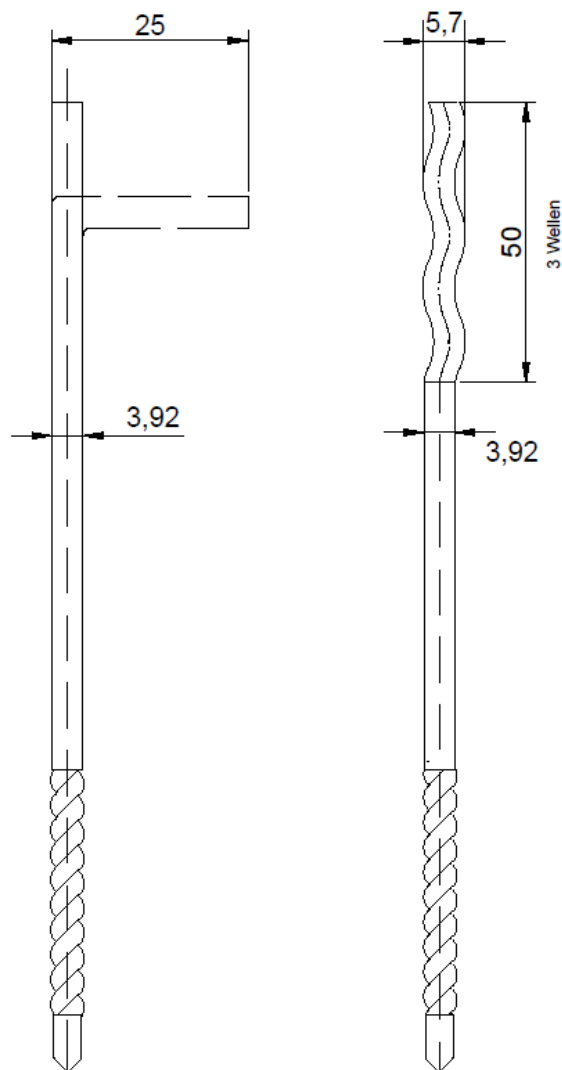
Drahtanker / Drahtanker mit Welle D 4mm
