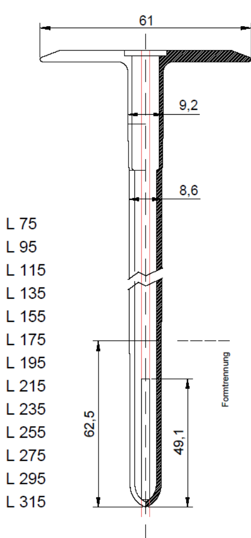
Dübelhülse
