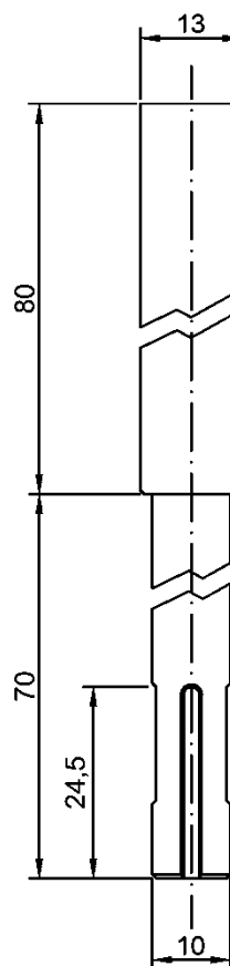
Einschlagadapter für Bohrhammer Anwendung für Drahtanker Ø5mm
