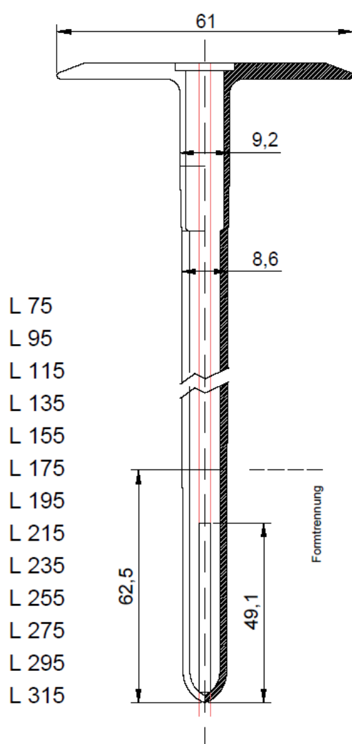
Dübelhülse
